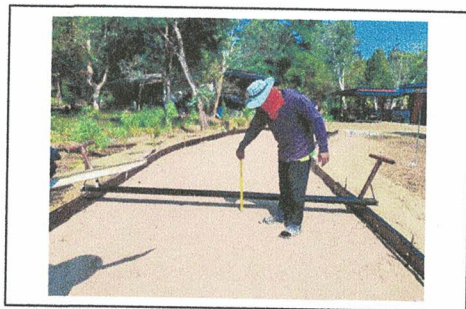
ก่อสร้างถนน คสล.สาย อบต.พัฒนา 1/1 หมู่ที่ 1
